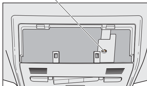
Betätigungsschraube zur Notbetätigung des elektrohydraulischen Aufstelldaches
